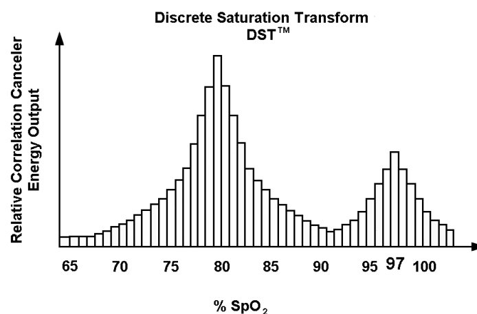
Fig. 80 DST™ Plot: Rauschunterdrückung als Funktion von SpO 2
