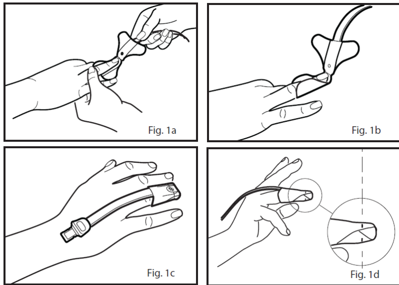
Fig. 19 RD SET Sensor Anwendung für Pädiatrie 10-50 kg
