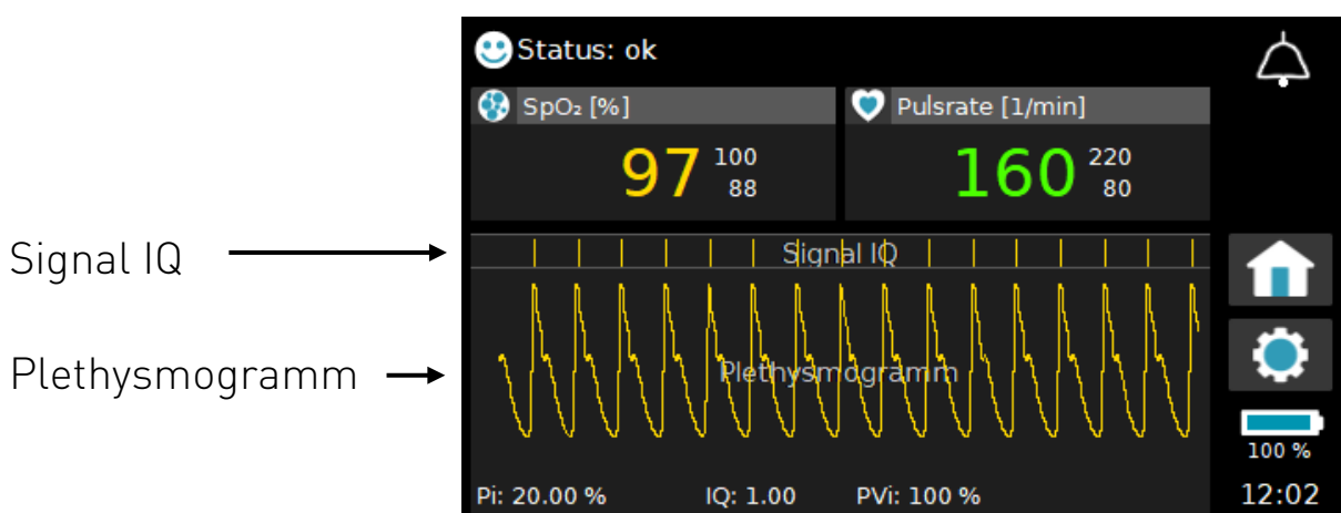
Fig. 40 Ansichten 3, SpO 2 und Pulsrate
